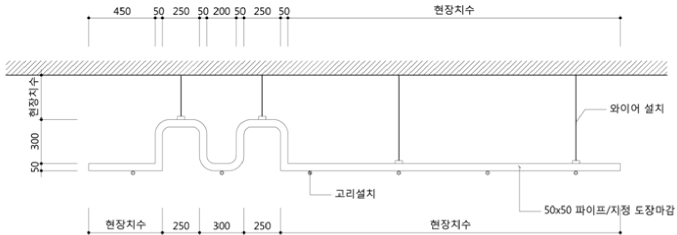
"M"-LINE 현수막 걸이 SCALE 1/20
